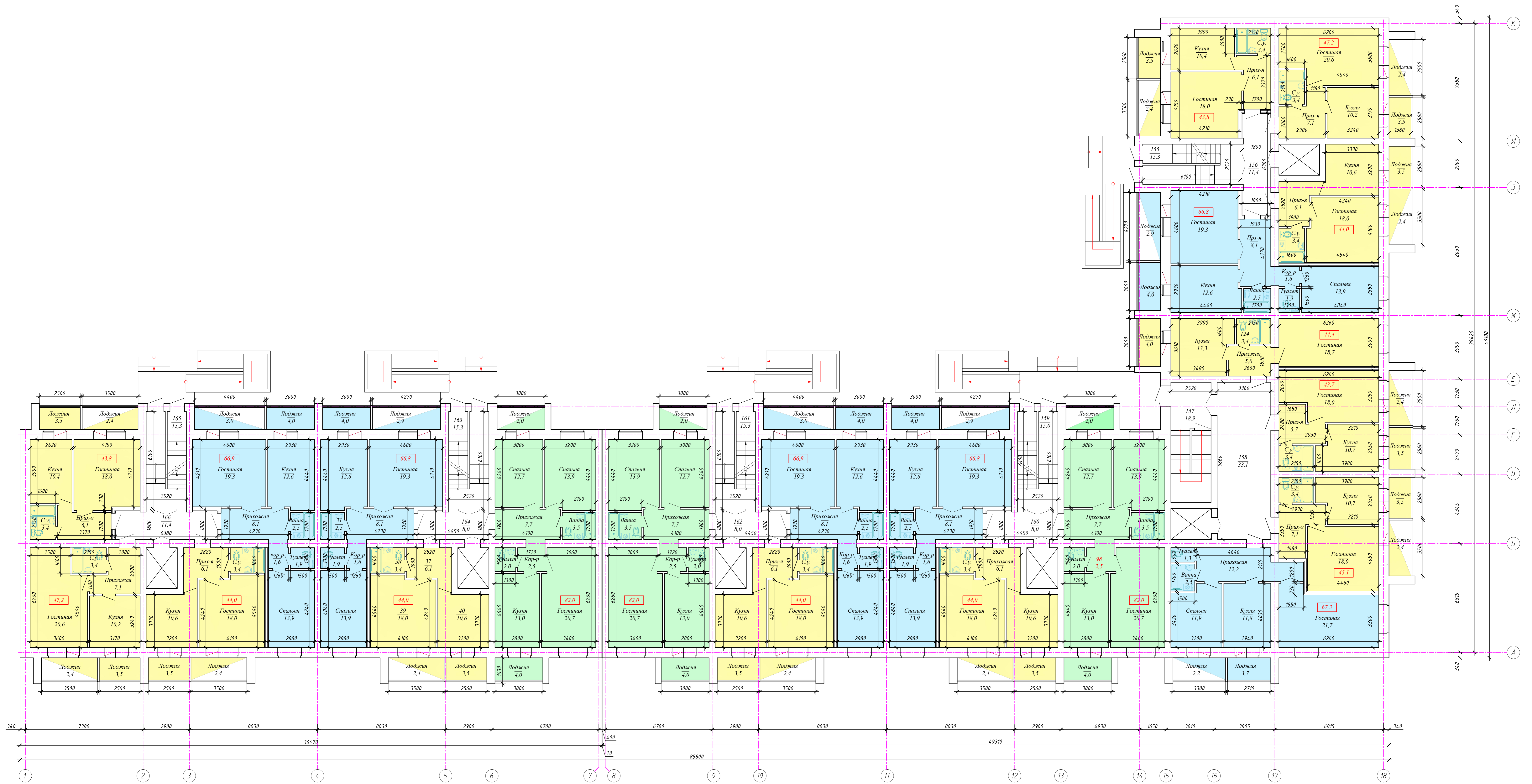
План первого этажа корпус 2
