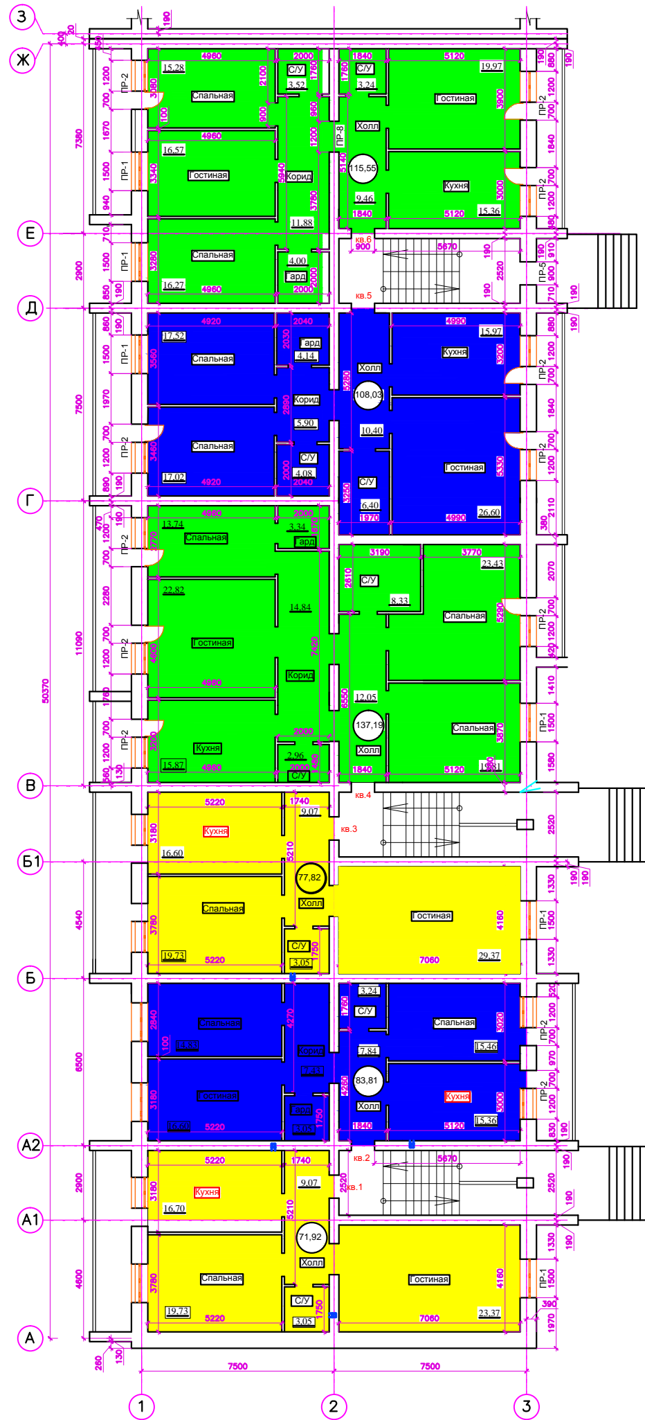
План первого этажа (М1:100)
