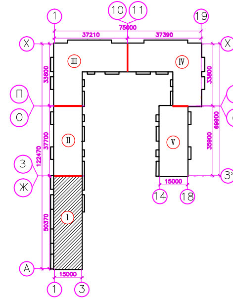
Схема здания
